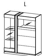
SI-KB2 (L, P) W: 1221, S: 1000, G: 440
