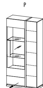
SI-W2 (L/P) W: 2071, S: 1000, G: 440
